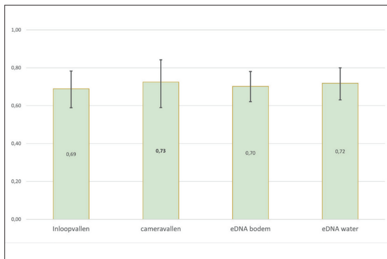
7a Gemiddeldetrefkans met 95 % betrouwbaarheidsinterval van alle onderzoeksmethoden.
